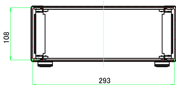
A-A ( 1 : 4.5 )
